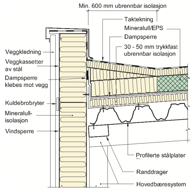
Fig. 10 Eksempel på avslutning mot langvegg av stålkonstruksjon.
