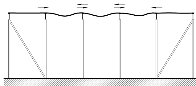
Fig. 4 Prinsskisse for membrankrefter (hengekabel)
