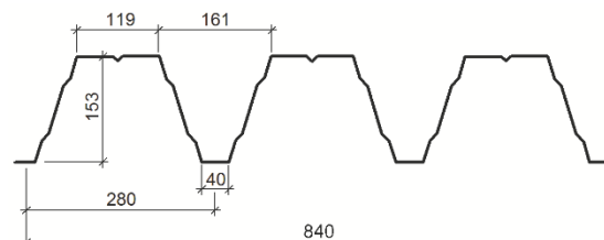
Fig. 2b Tata Steel plateprofil SAB 153/840 for stålplatetak med brannmotstand R15 – R60
