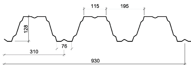
Fig. 2a Tata Steel plateprofil 128R.930 for stålplatetak med brannmotstand R15 – R60
