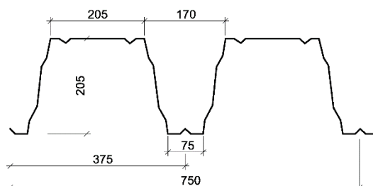
Fig. 3c Tata Steel plateprofil SAB 200R/750 for stålplatetak med brannmotstand R15 – R60
