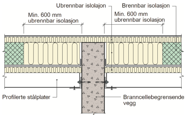
Fig. 9 Prinsipp for tilslutning mellom branncellebegrensende vegg og tak. Profiler vinkelrett på vegg. Boltene som holder opplegget for stålplatene skal være mutterbolter med store skiver, ikke gjennomgående.
